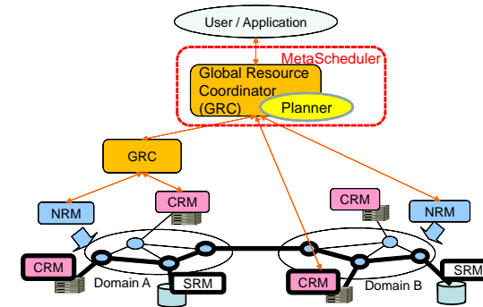
図 1 資源管理システム RMS の概要
