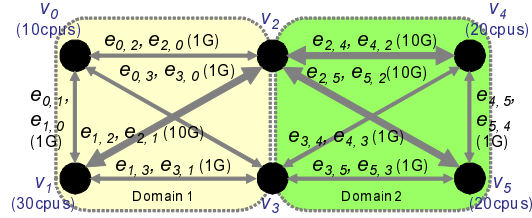
図3 資源グラフ
