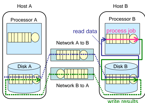
図3 データグリッドコンピューティングにおけるBricksシミュレーションの流れ. Fig.3 Bricks simulation steps for Data intensive computing.
